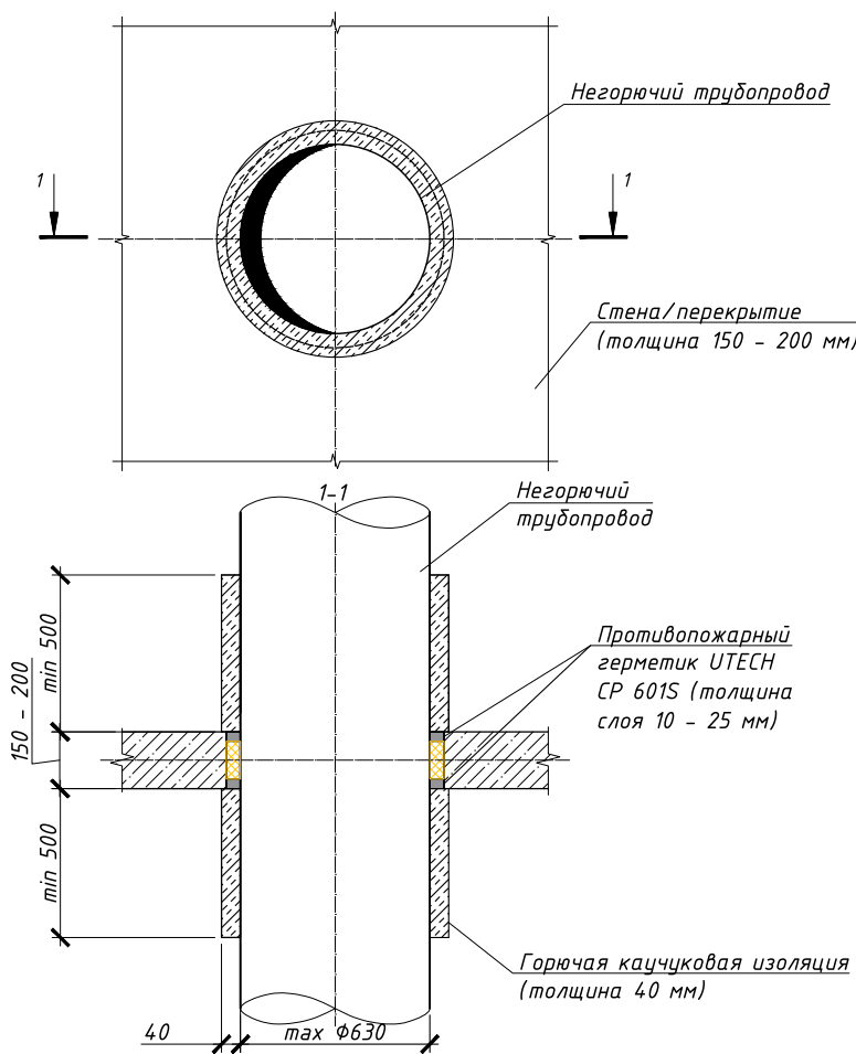
Узел пересечения ограждающих конструкций негорючими трубопроводами с применением противопожарного герметика UTECH CP601S
